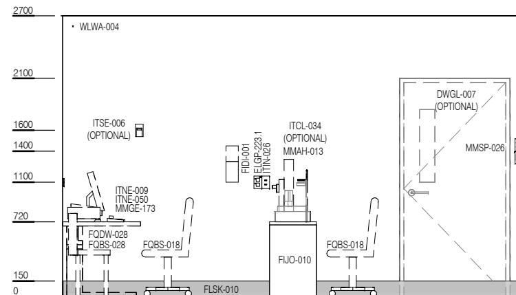
ELEVATION 2
