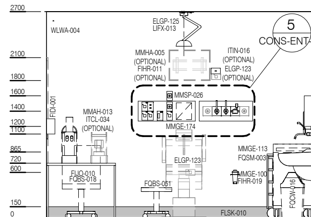
ELEVATION 3
