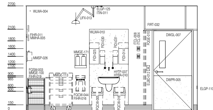
ELEVATION 4
