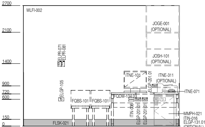
ELEVATION 1
