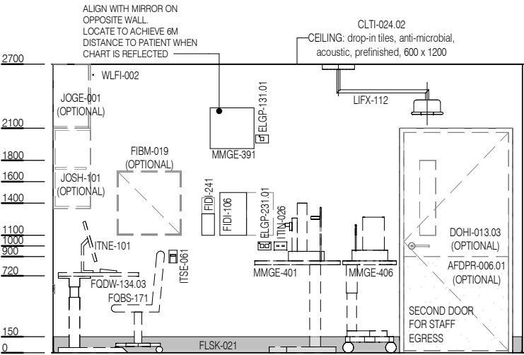
ELEVATION 2
