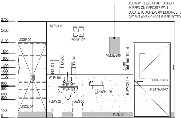
ELEVATION 4
