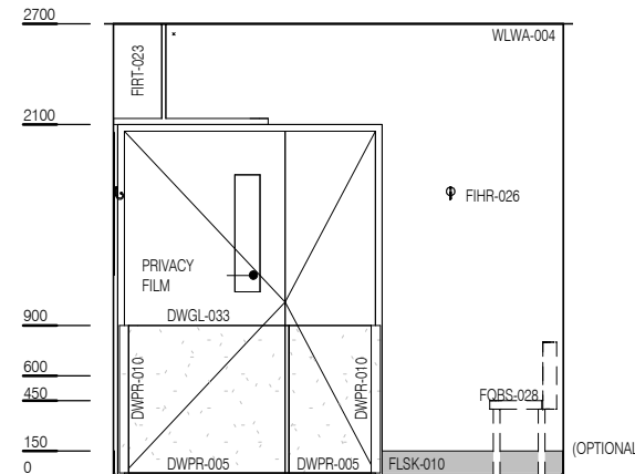
ELEVATION 3
