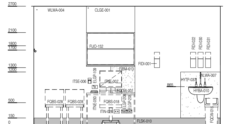
ELEVATION 4
