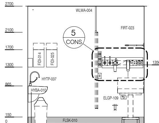
ELEVATION 1
