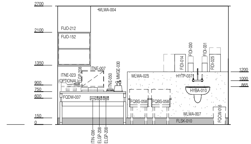
ELEVATION 4
