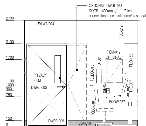
ELEVATION 3
