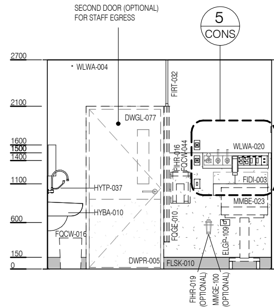
ELEVATION 1
