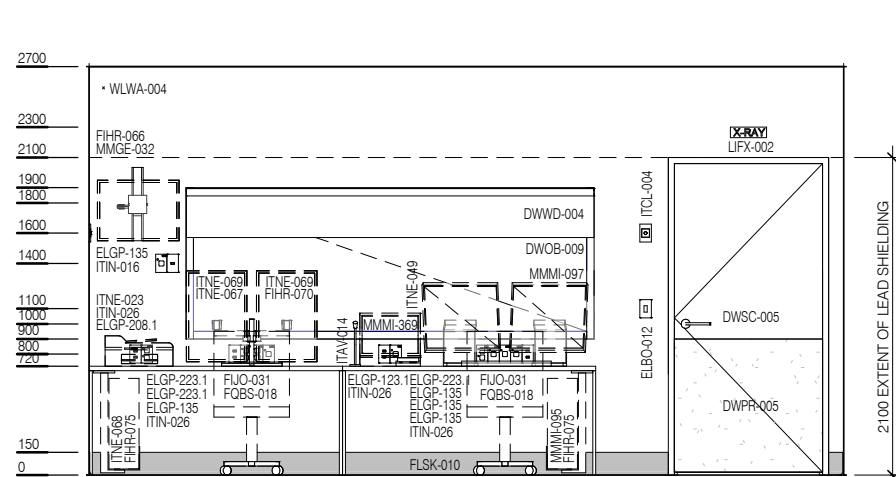
ELEVATION 2
