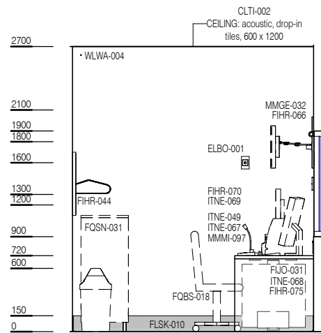
ELEVATION 1
