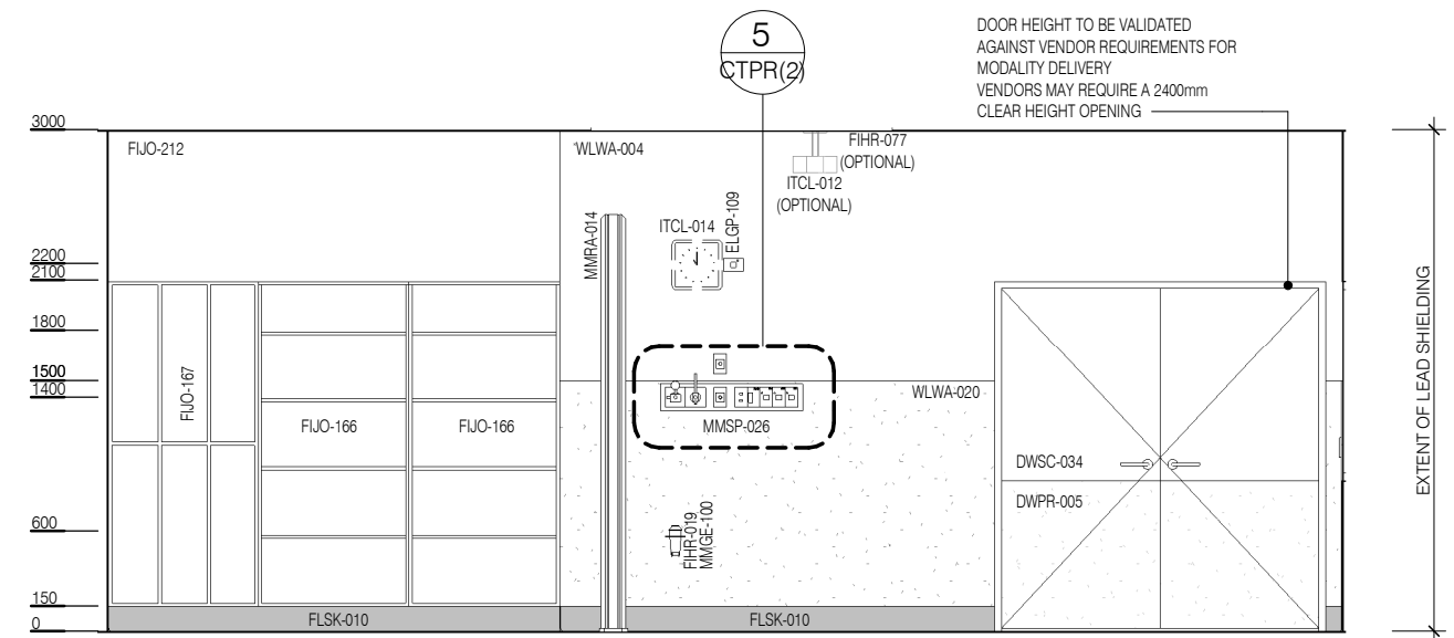
ELEVATION 2
