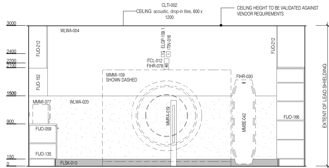
ELEVATION 1
