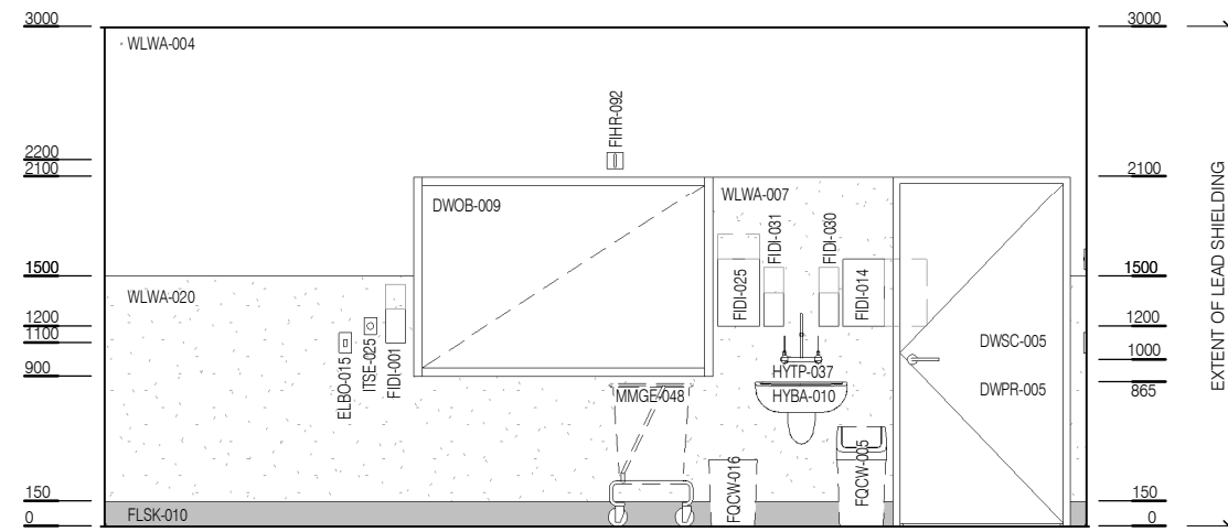
ELEVATION 3
