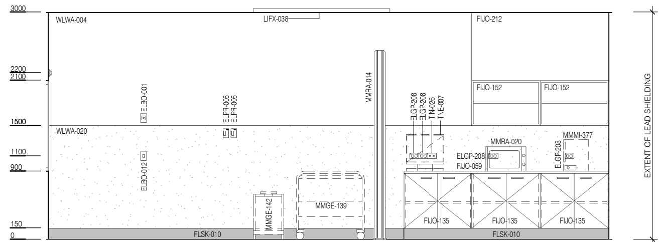
ELEVATION 4
