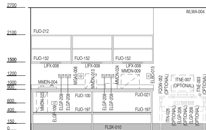
ELEVATION 2
