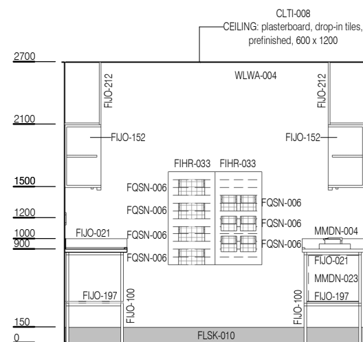
ELEVATION 1
