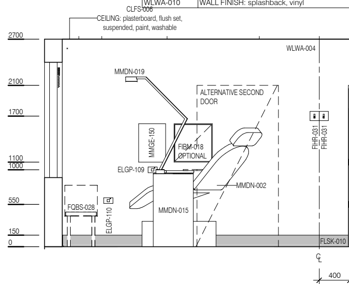
ELEVATION 2
