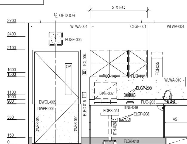
ELEVATION 3
