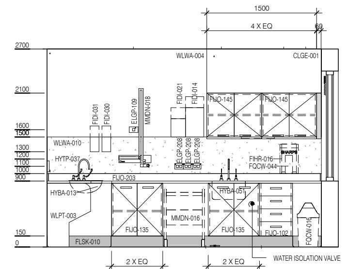
ELEVATION 4
