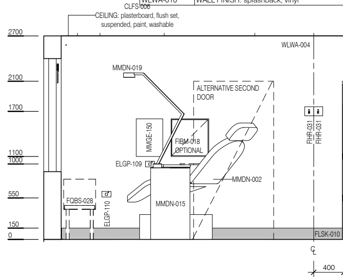
ELEVATION 2
