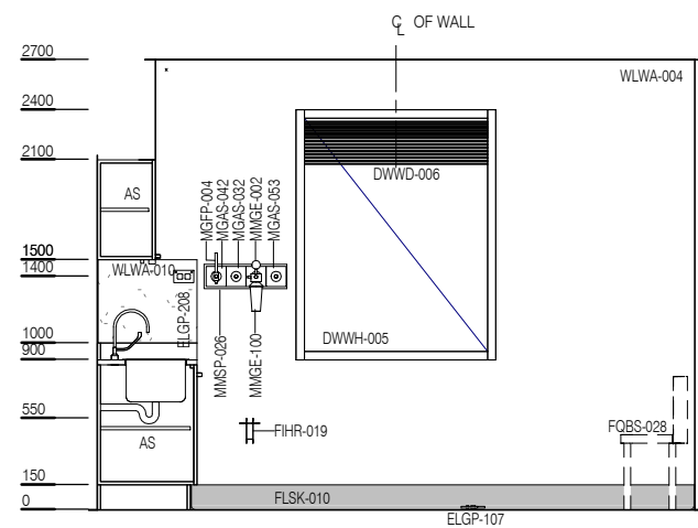
ELEVATION 1
