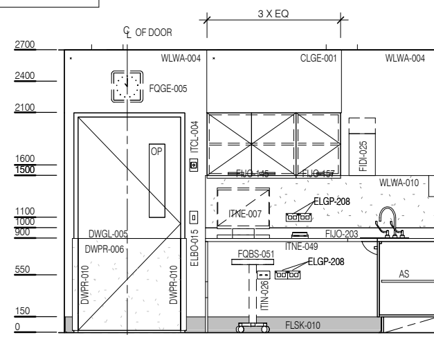
ELEVATION 3
