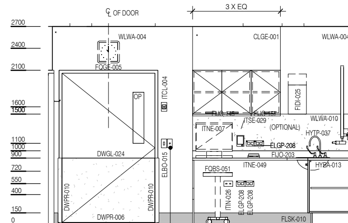
ELEVATION 3
