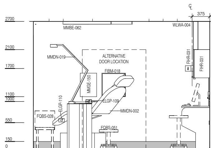
ELEVATION 2
