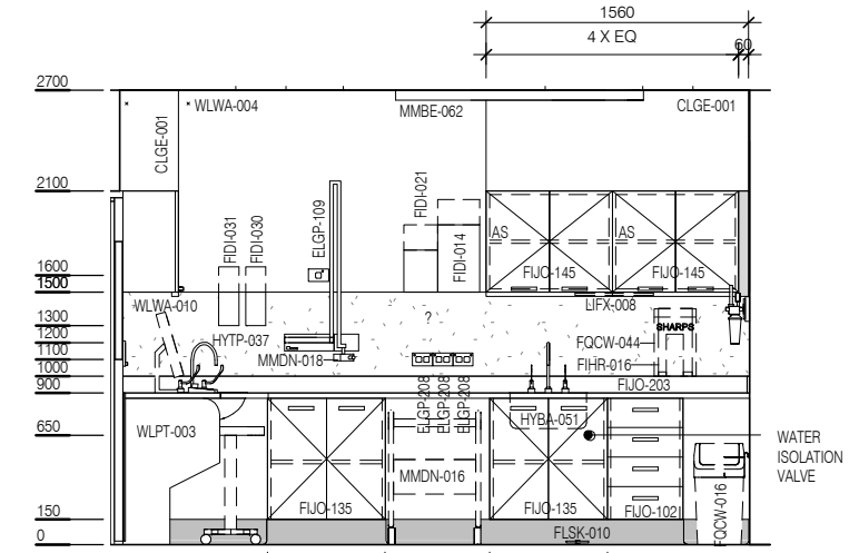
ELEVATION 4
