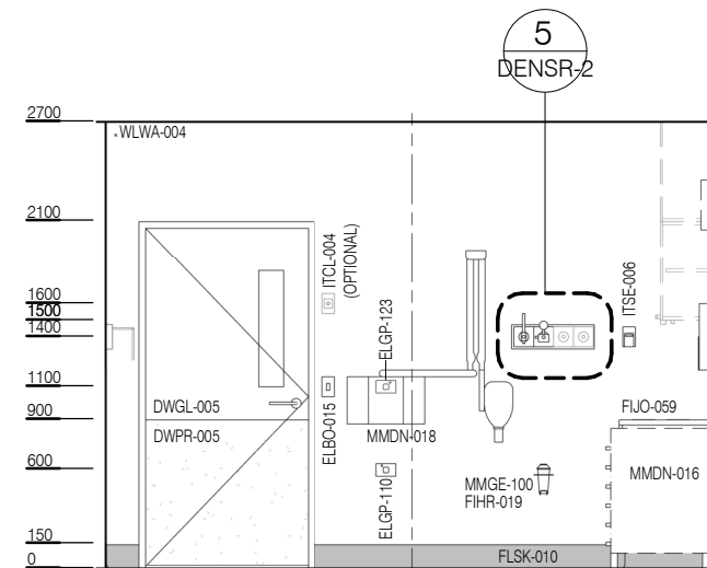
ELEVATION 3
