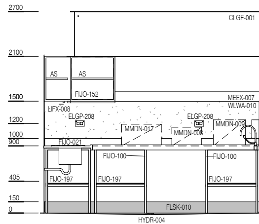
ELEVATION 1
