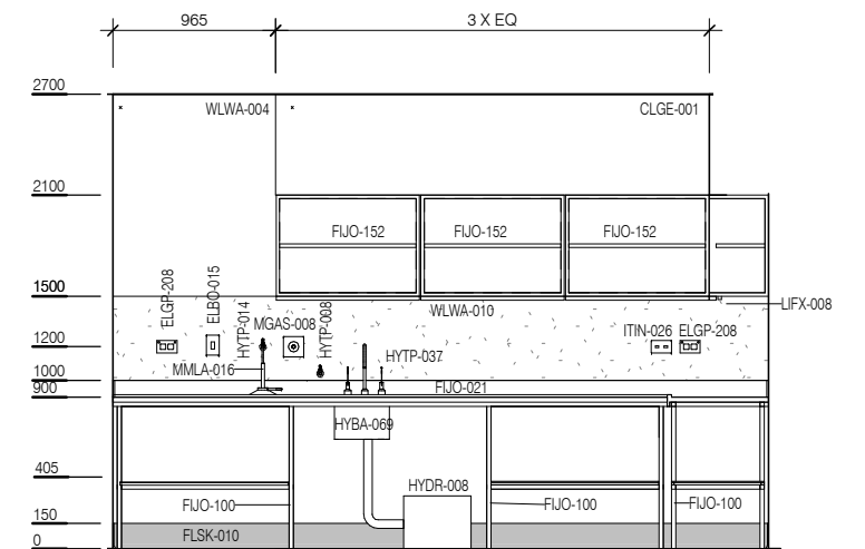
ELEVATION 4
