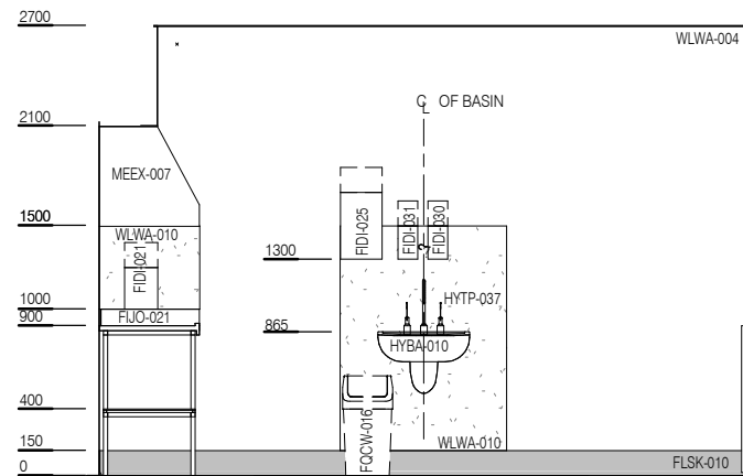
ELEVATION 2
