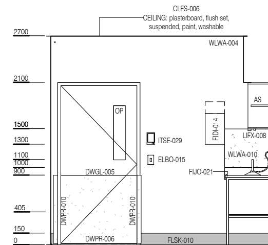
ELEVATION 3
