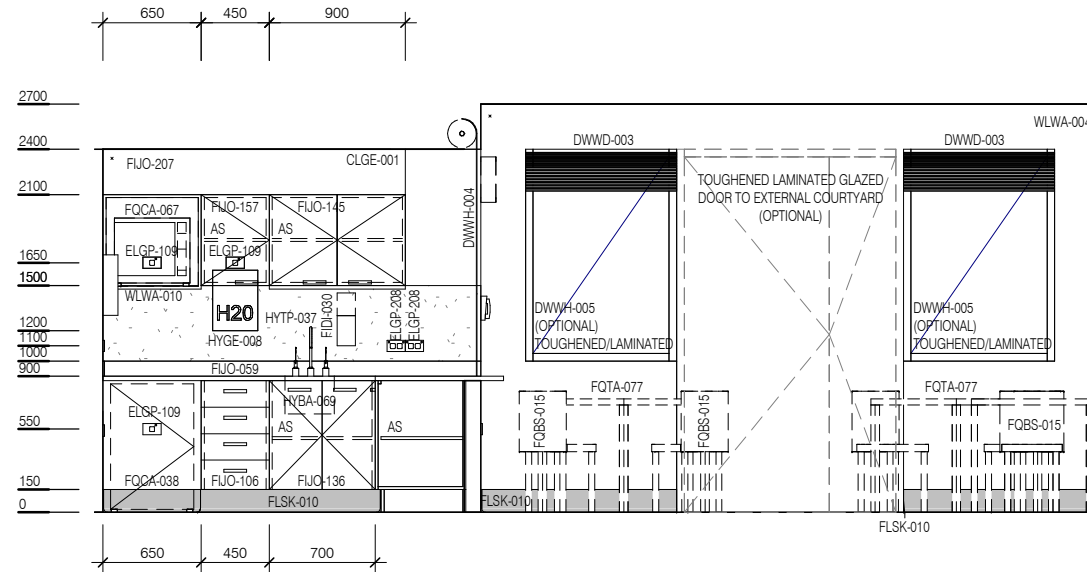
ELEVATION 1
