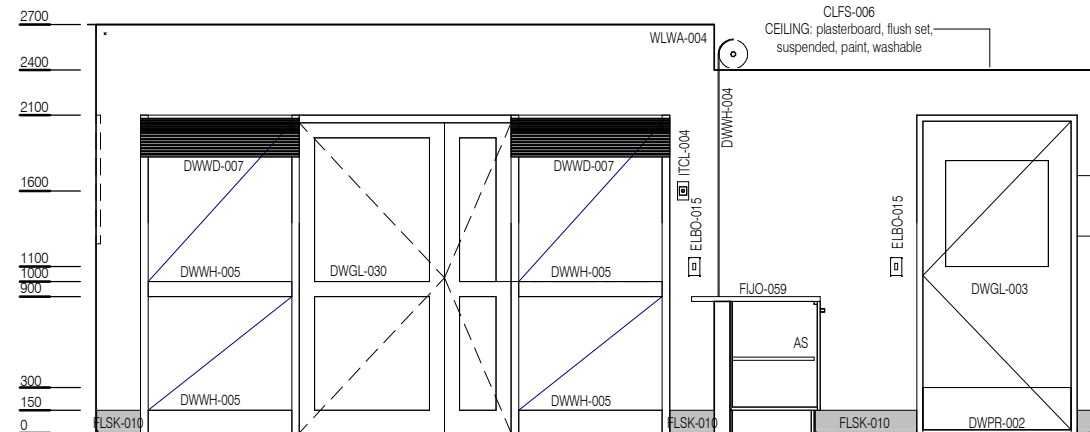
ELEVATION 3
