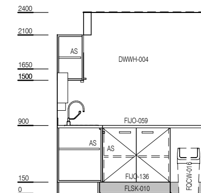
ELEVATION 5
