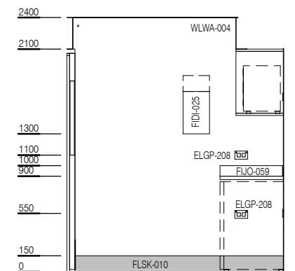
ELEVATION 6
