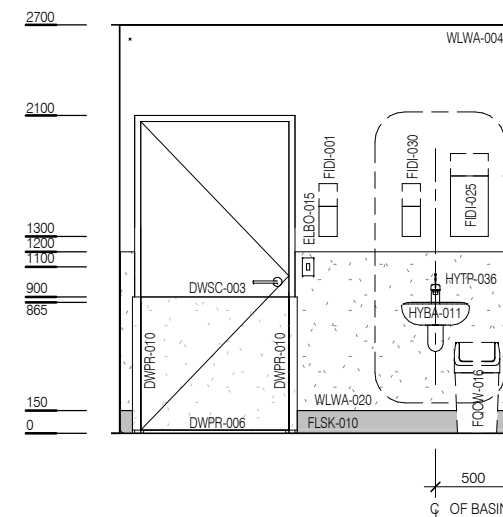
ELEVATION 3
