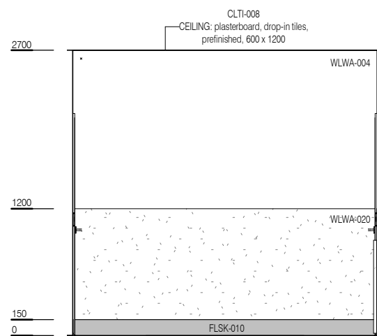
ELEVATION 2
