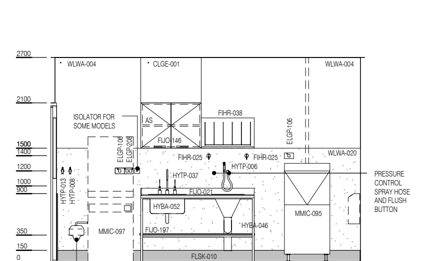
ELEVATION 4
