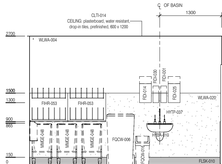
ELEVATION 2
