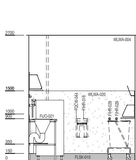
ELEVATION 1
