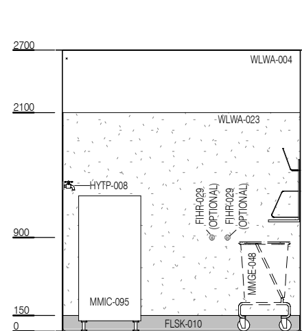
ELEVATION 1
