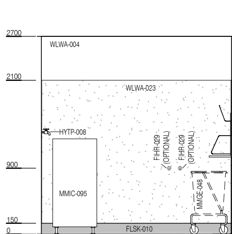
ELEVATION 1
