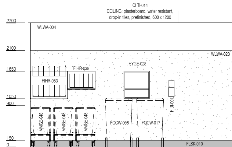
ELEVATION 2
