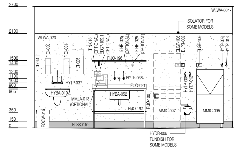
ELEVATION 4
