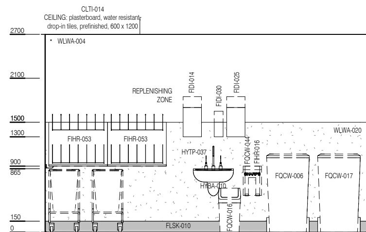
ELEVATION 2
