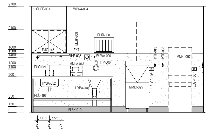
ELEVATION 4
