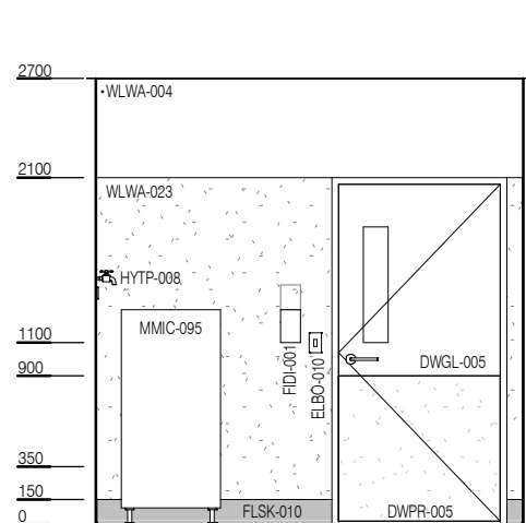
ELEVATION 1
