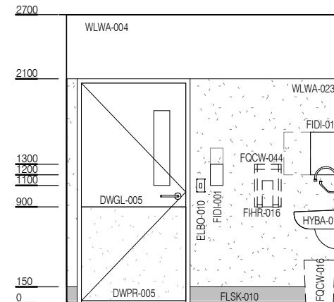
ELEVATION 3
