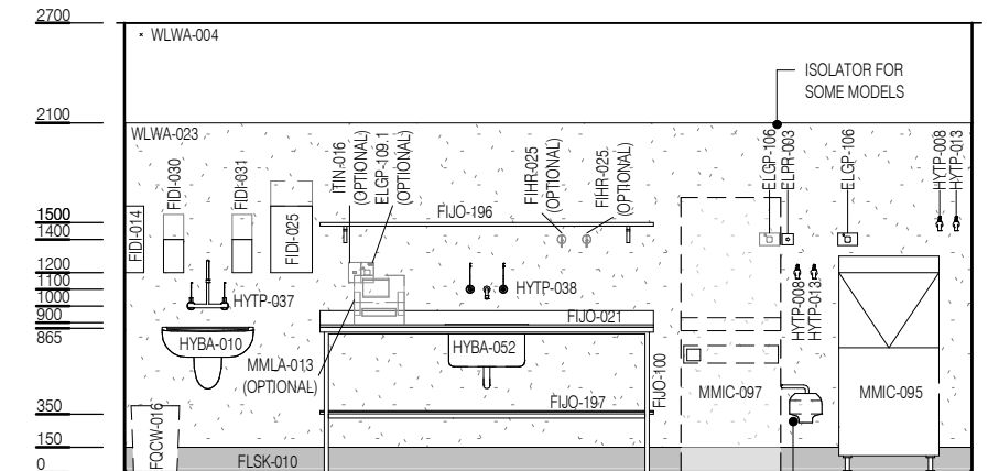
ELEVATION 4
