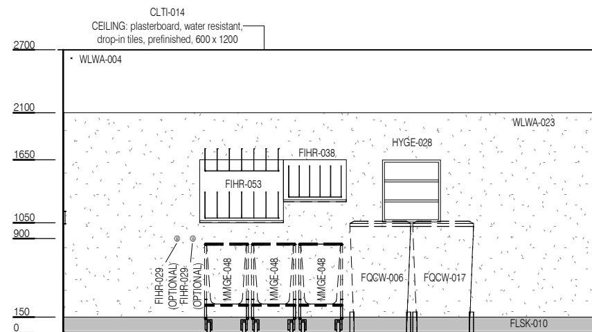
ELEVATION 2
