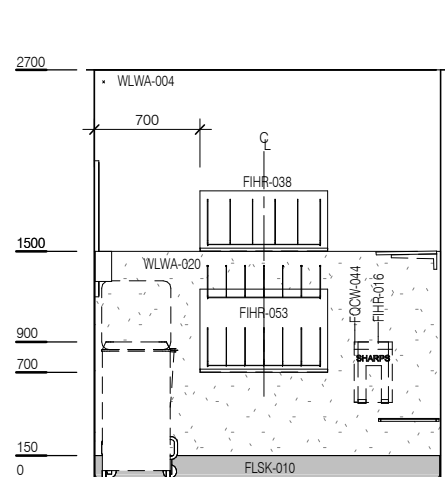
ELEVATION 1
