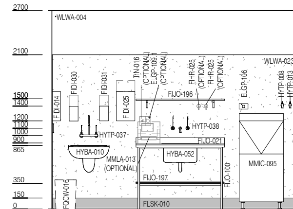
ELEVATION 4
