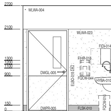
ELEVATION 3
