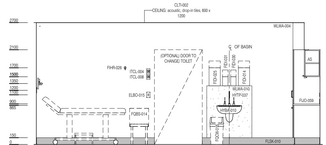
ELEVATION 2
