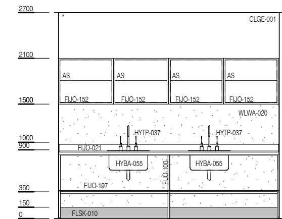
ELEVATION 4
