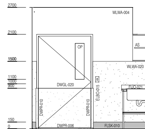
ELEVATION 3
