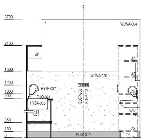
ELEVATION 1
