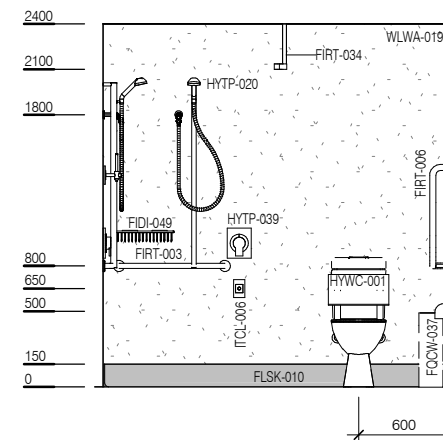
ELEVATION 3
