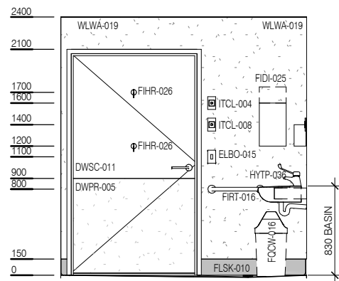
ELEVATION 1
