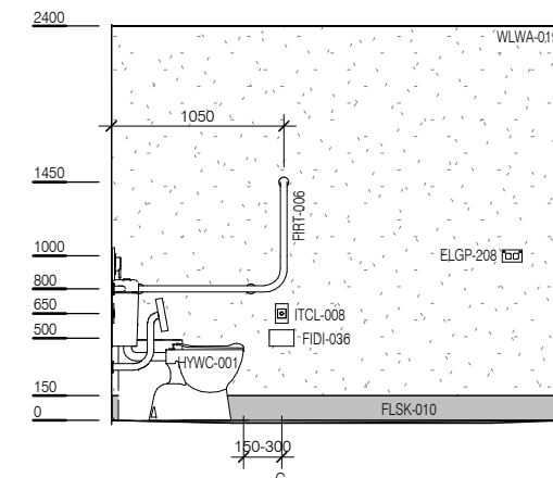
ELEVATION 4
