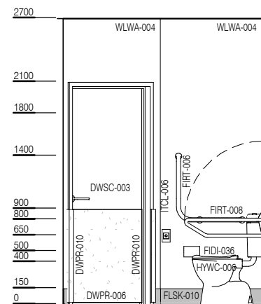
ELEVATION 2
