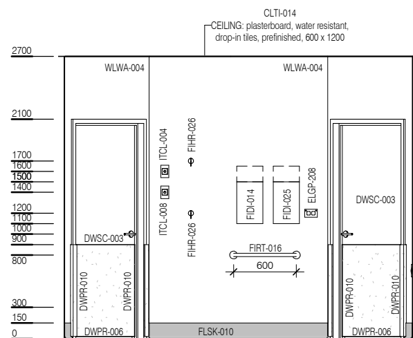
ELEVATION 1
