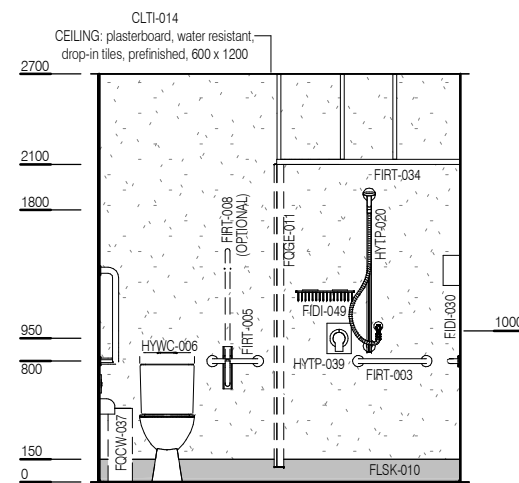
ELEVATION 2
