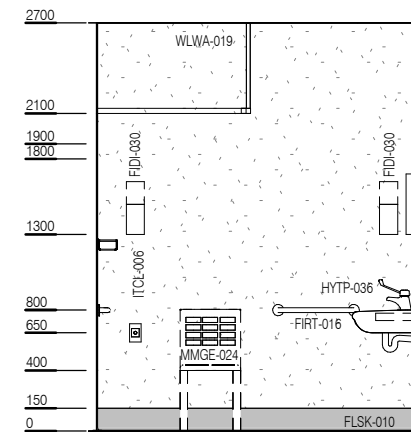
ELEVATION 3
