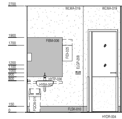
ELEVATION 4
