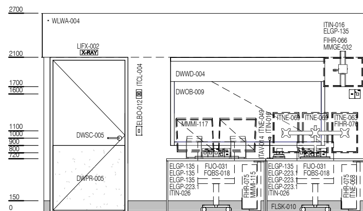
ELEVATION 2
