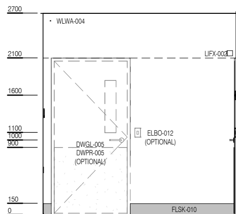
ELEVATION 1
