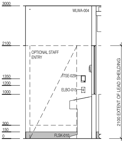
ELEVATION 6
