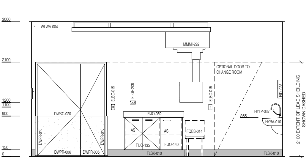
ELEVATION 3
