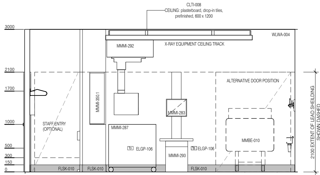
ELEVATION 1
