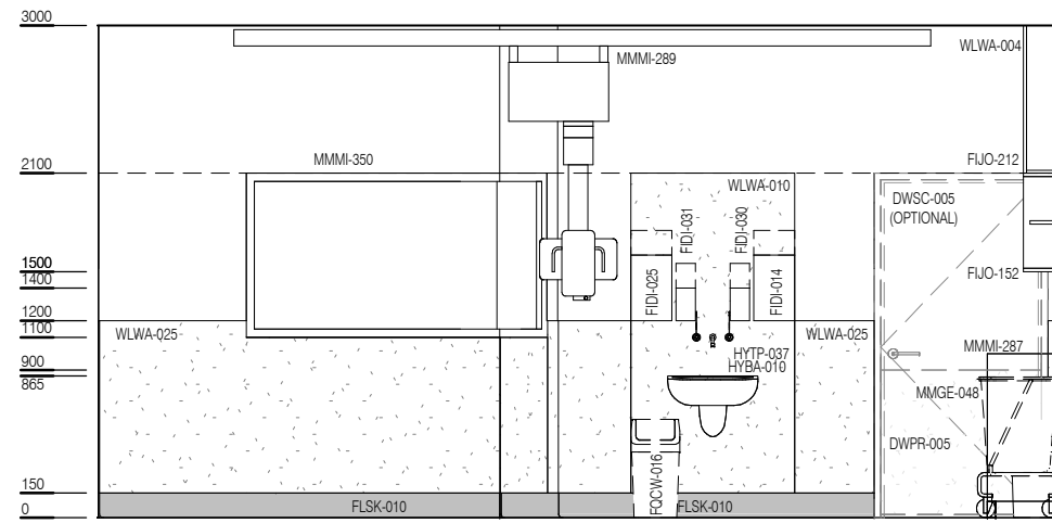
ELEVATION 3
