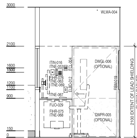
ELEVATION 6
