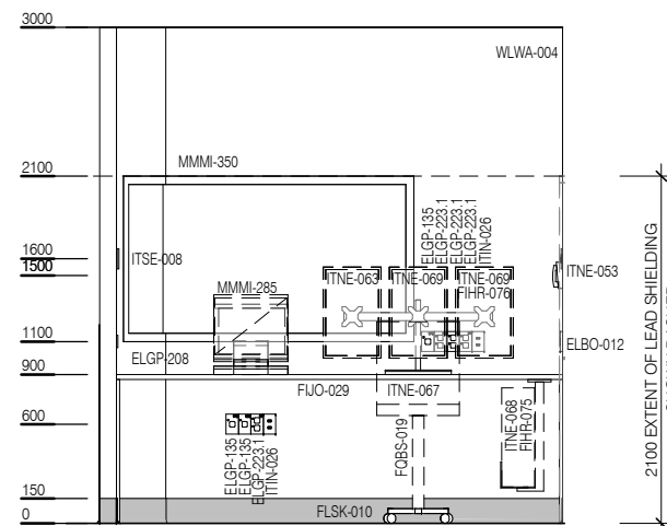
ELEVATION 5
