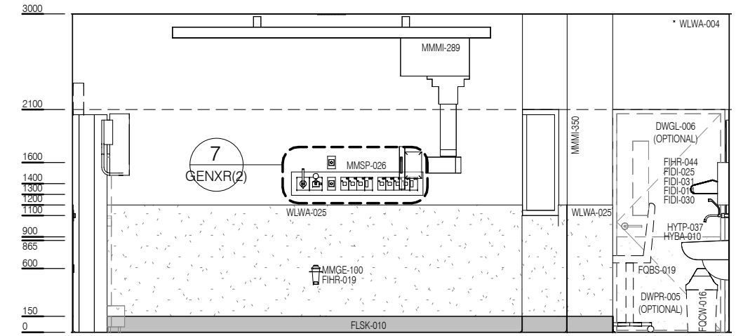
ELEVATION 2
