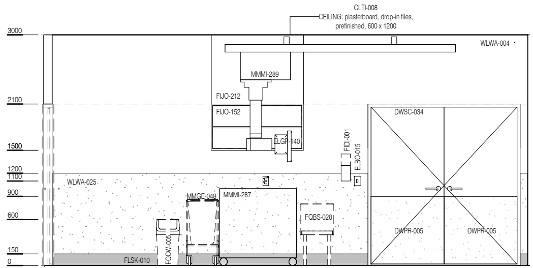
ELEVATION 4
