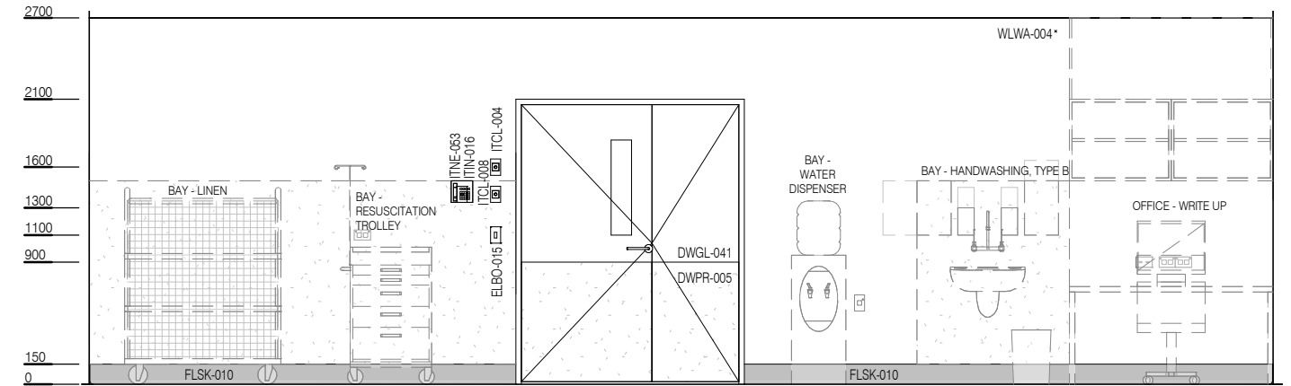
ELEVATION 3
