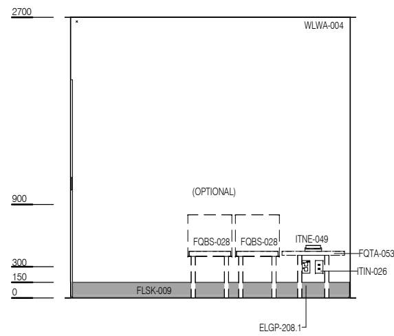
ELEVATION 1
