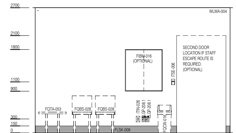
ELEVATION 4
