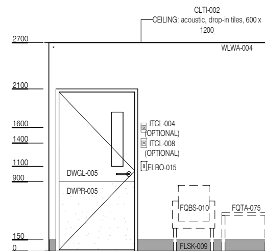
ELEVATION 3
