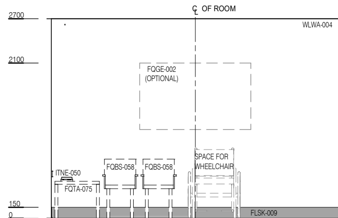
ELEVATION 2
