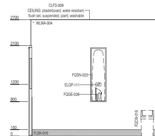
ELEVATION 4
