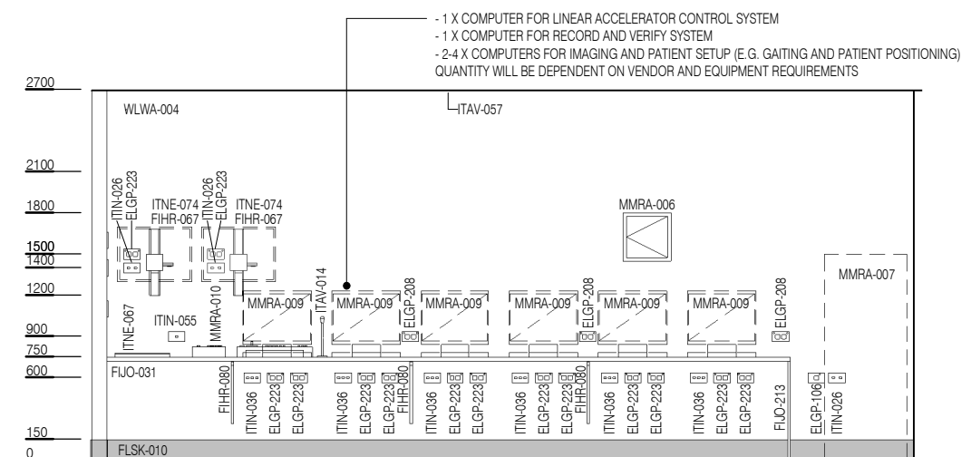
ELEVATION 4
