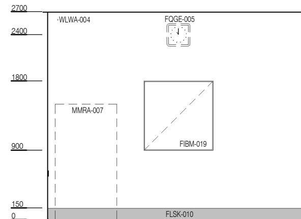
ELEVATION 1
