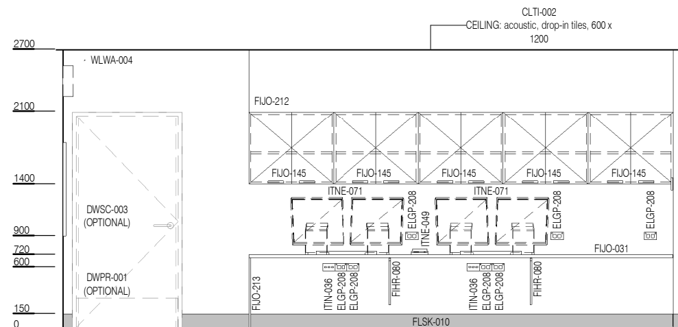
ELEVATION 2
