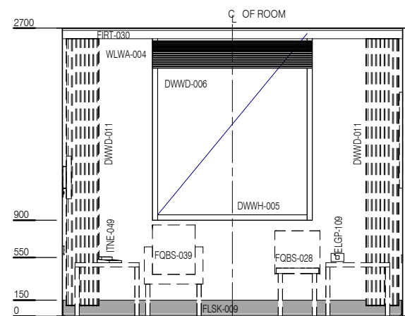
ELEVATION 1
