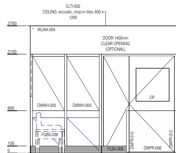
ELEVATION 3
