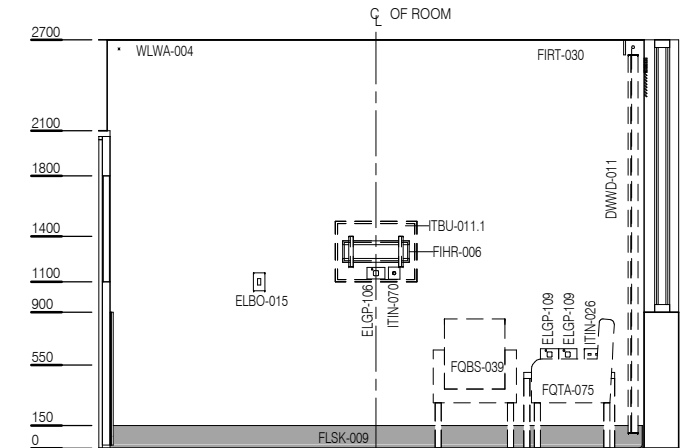
ELEVATION 4
