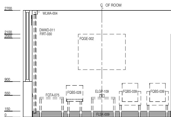
ELEVATION 2
