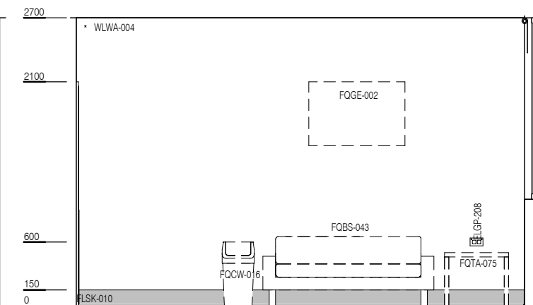
ELEVATION 4
