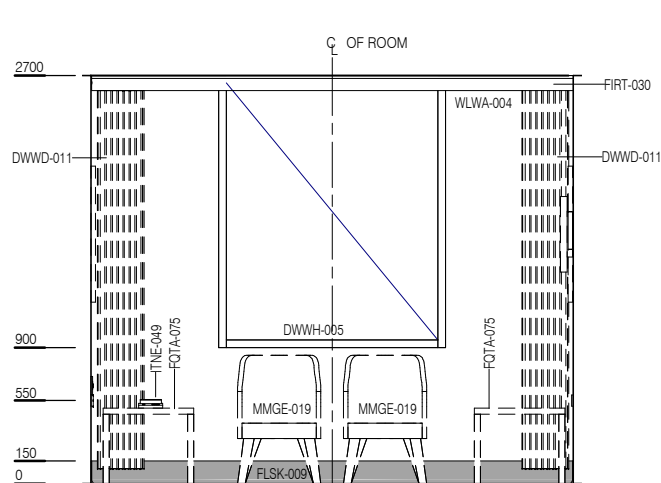
ELEVATION 1
