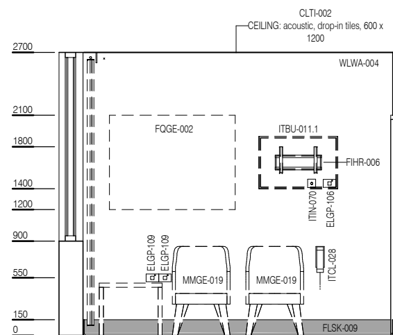
ELEVATION 2
