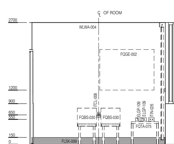
ELEVATION 4
