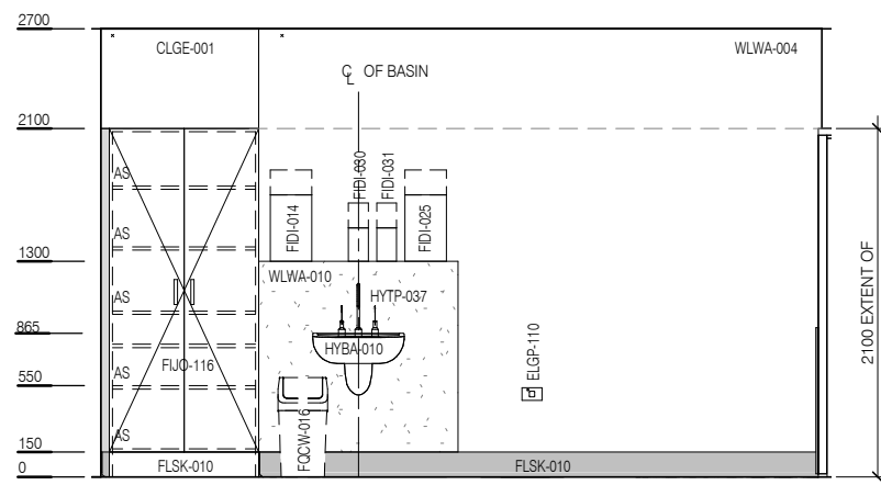
ELEVATION 2
