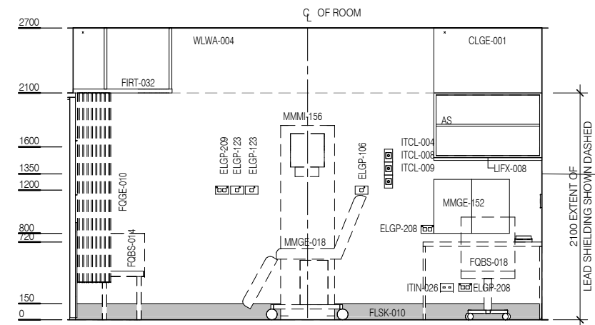
ELEVATION 4
