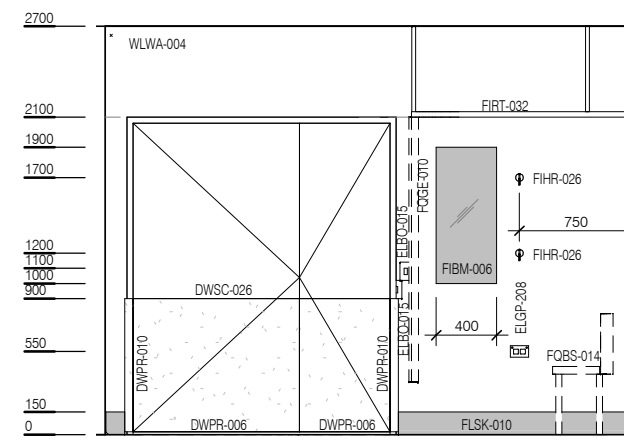
ELEVATION 3
