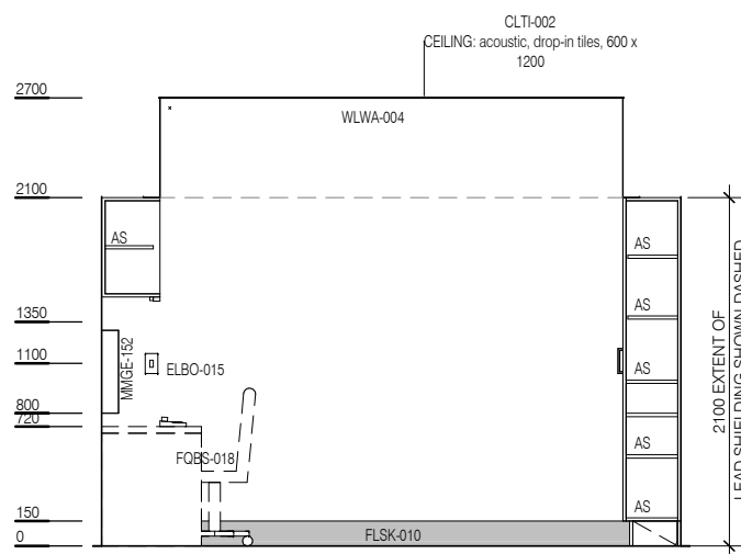
ELEVATION 1
