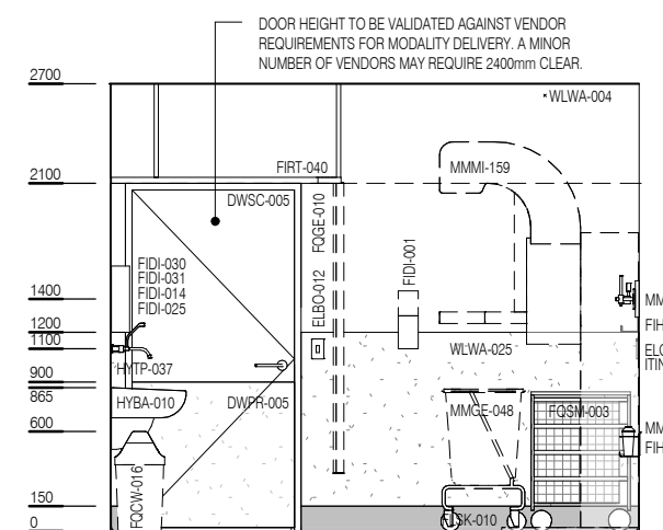
ELEVATION 3
