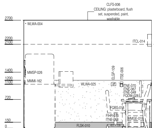
ELEVATION 1
