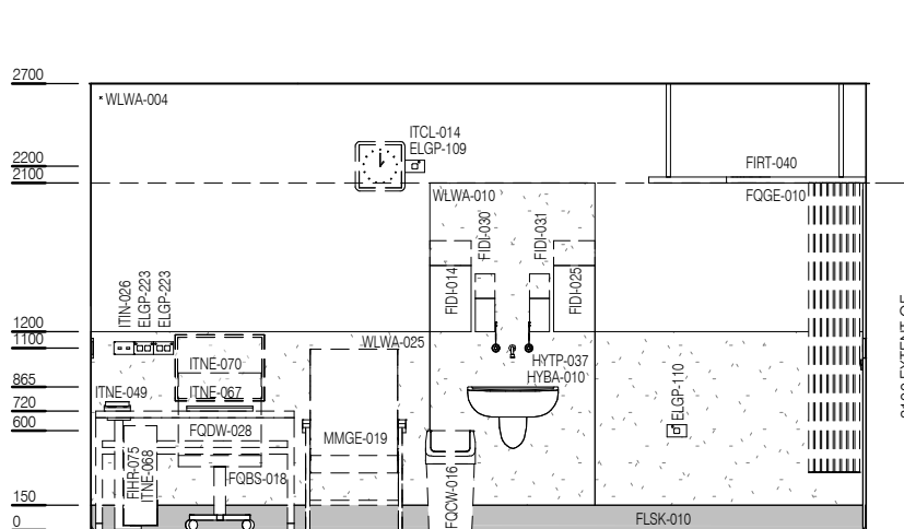
ELEVATION 2
