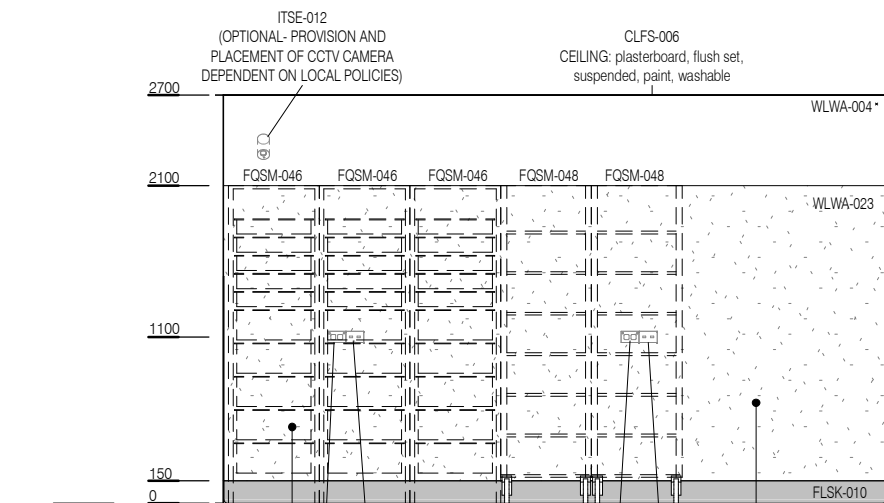
ELEVATION 2
