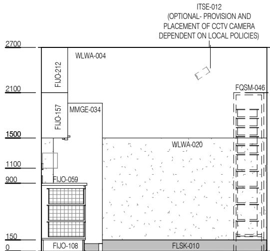
ELEVATION 1
