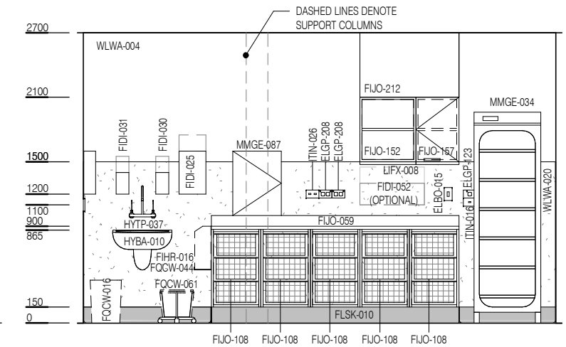
ELEVATION 4
