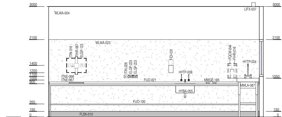
ELEVATION 4
