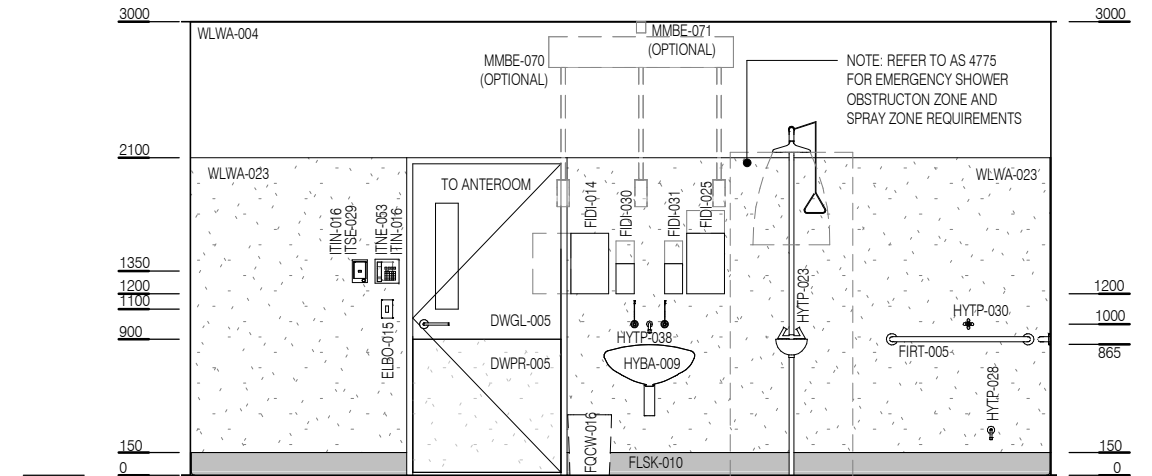
ELEVATION 2
