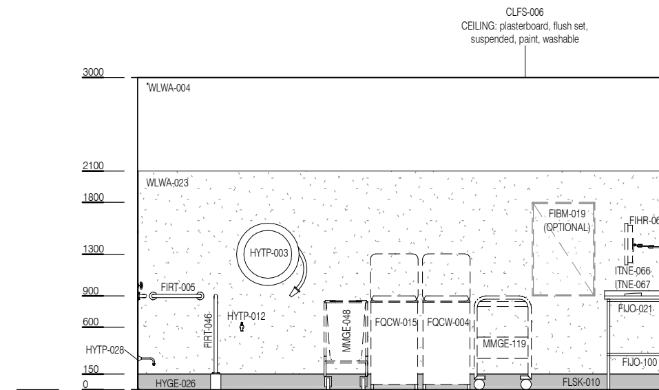
ELEVATION 3
