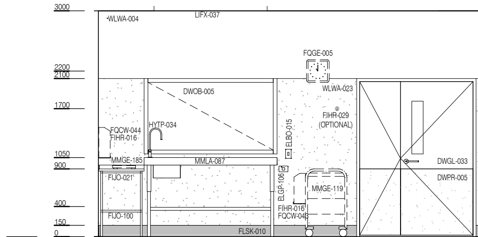
ELEVATION 1
