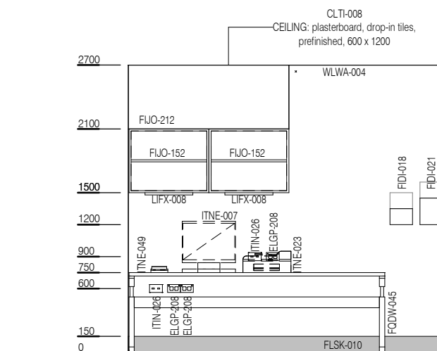
ELEVATION 2
