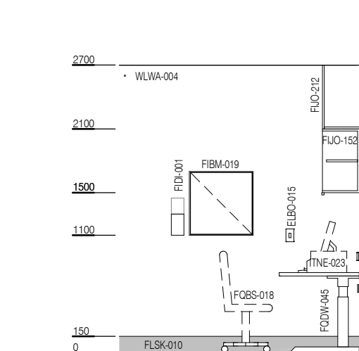
ELEVATION 1
