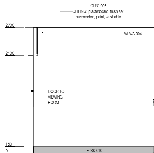
ELEVATION 1
