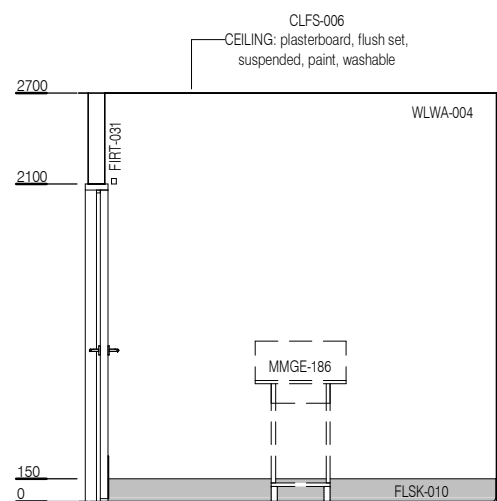
ELEVATION 1
