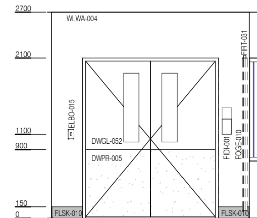
ELEVATION 3
