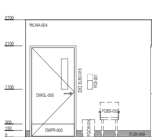
ELEVATION 1
