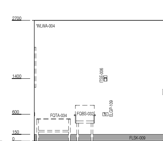
ELEVATION 4
