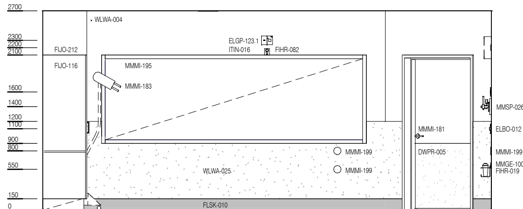
ELEVATION 3
