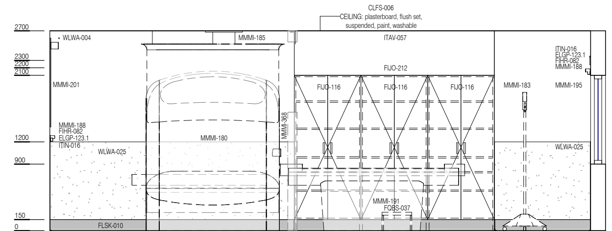
ELEVATION 2
