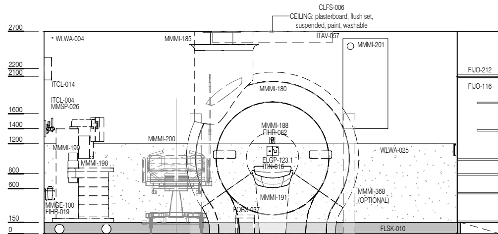
ELEVATION 1
