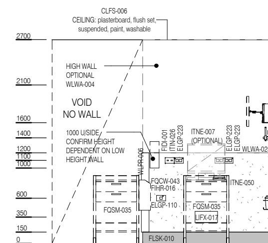
ELEVATION 3
