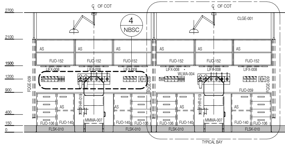
ELEVATION 1
