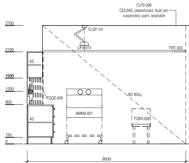
ELEVATION 2
