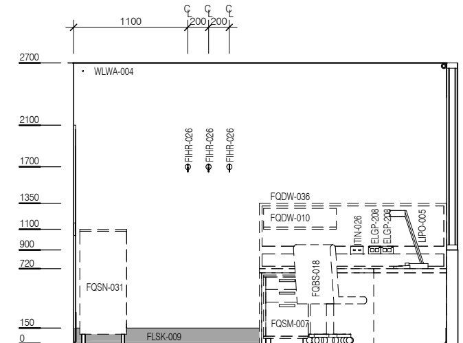
ELEVATION 4
