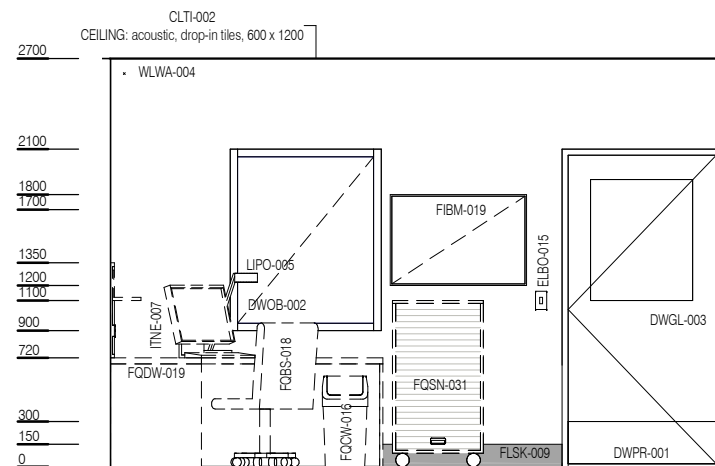
ELEVATION 3
