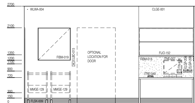
ELEVATION 4
